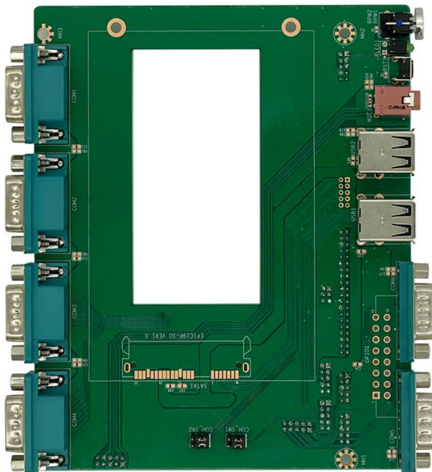
MB35-600U VER1.0 配套的 IO 板
